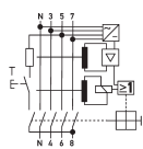
Schaltungsbeispiel Fehlerstromschutzschalter DFS 4 063-4/0,03-F EV
