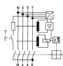
Schaltungsbeispiel Fehlerstromschutzschalter DFS 4 063-4/0,03-A EV HD
