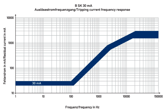
Diagramme Fehlerstromschutzschalter DFS 4 063-4/0,03-B SK R HD
