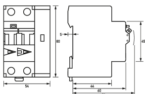
Maßzeichnung Fehlerlichtbogen-Schutzeinrichtungen DAFDD 1 B16/0,01/2-A
