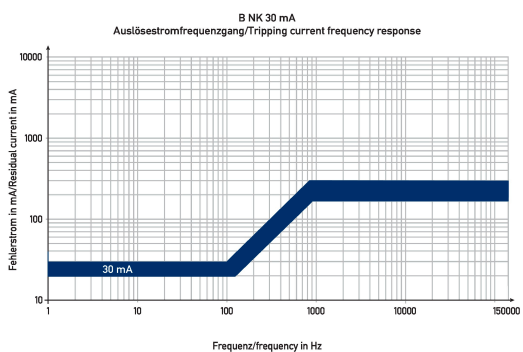
Diagramme Fehlerstromschutzschalter DFS 4 063-4/0,03-B NK V500
