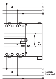
Schaltungsbeispiel Fehlerstromschutzschalter DRCCB 5 STR 063-4/0,03-A
