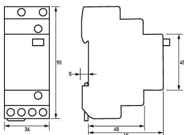
Maßzeichnung Stromstoßschalter (Fernschalter) RS 230-002
