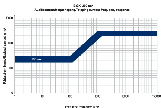
Diagramme Fehlerstromschutzschalter DFS 4 040-4/0,30-B SK R
