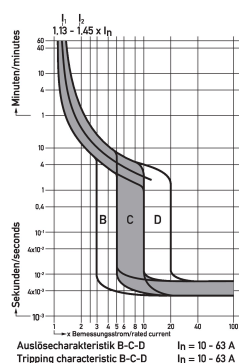
Diagramme Leitungsschutzschalter DLS 6i C10-1
