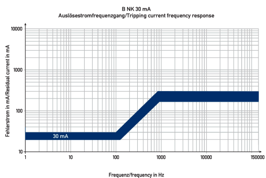
Diagramme Fehlerstromschutzschalter DFS 4 125-4/0,03-B NK
