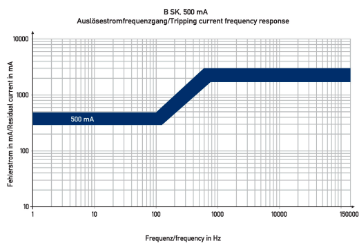
Diagramme Fehlerstromschutzschalter DFS 4 063-4/0,50-B SK
