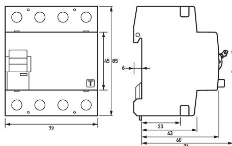
Maßzeichnung Fehlerstromschutzschalter DFS 4 040-4/0,30-PV
