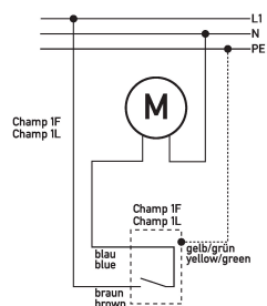
Schaltungsbeispiel Schwimmerschalter Champ 1 GS-L 03 m
